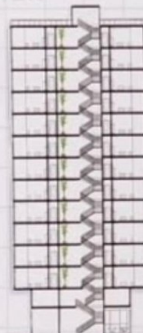
Section A-A 1/200
