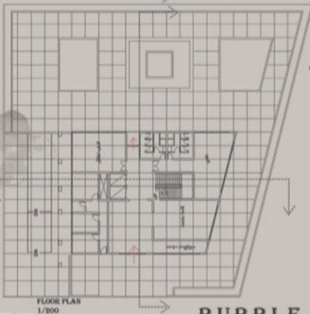
PLAN 2 05/10/10/10 1/200
